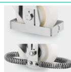
Retningslås Hjul i 4680-serien kan festes med både en kort og lang (XL) retningslås. Målene finner du på hjemmesiden vår.
